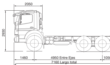
DIMENSIONES (mm)
